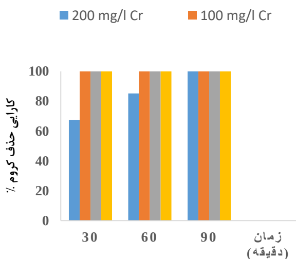
نمودار ۶: تاثیر غلظت اولیه کروم شش ظرفیتی بر کارایی حذف (شدت جریان 100 \text{ mA} ، \text{pH}=3 ، غلظت اسید تیوگلیکولیک 0.04 \text{ cc/250cc} ، \text{NaCl} : 50 \text{ mg/l} )
