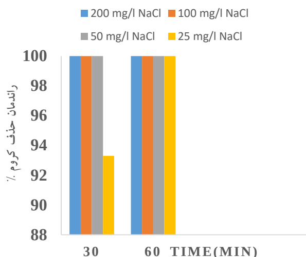
شکل ۷: نمودار تاثیر غلظت حمایت کننده الکترولیتی بر روی حذف کروم شش ظرفیتی (غلظت کروم: 100 \text{ mg/L} ، شدت جریان 100 \text{ mA} ، \text{pH}=3 ، غلظت اسید تیوگلیکولیک 0.04 \text{ cc/250cc} )
