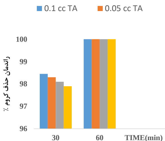
شکل ۴: نمودار تاثیر غلظت اسید تیوگلیکولیک اسید بر روی حذف کروم شش ظرفیتی (غلظت کروم: ۱۰۰ mg/L، شدت جریان ۱۰۰ mA، pH ۳، ۵۰ mg/L NaCl)
