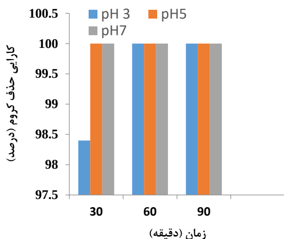
شکل ۲: نمودار تاثیر pH بر روی حذف کروم شش ظرفیتی در فرایند الکتروشیمی
